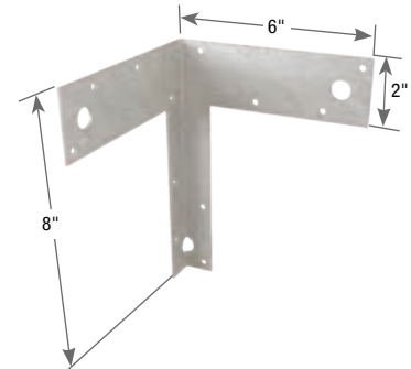
KSCT68
