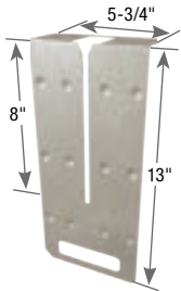
FWHL-T
