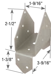
RT6
