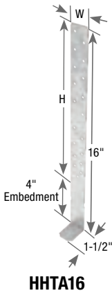
HHTA16
