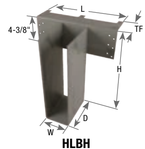
HLBH
