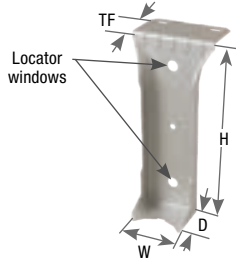
PHG26
