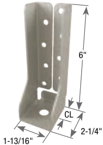
DTB-TZ
