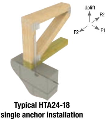
HTA24-18
