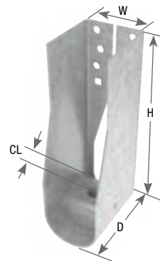
S/PHD4
