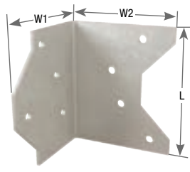
JA3
