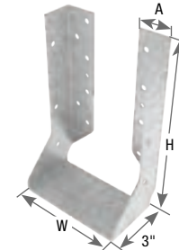
HDQIF
